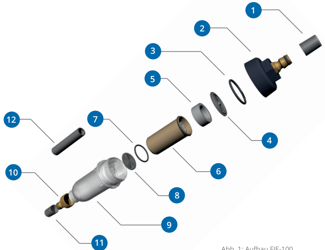
Abb. 1: Aufbau FIE-100
